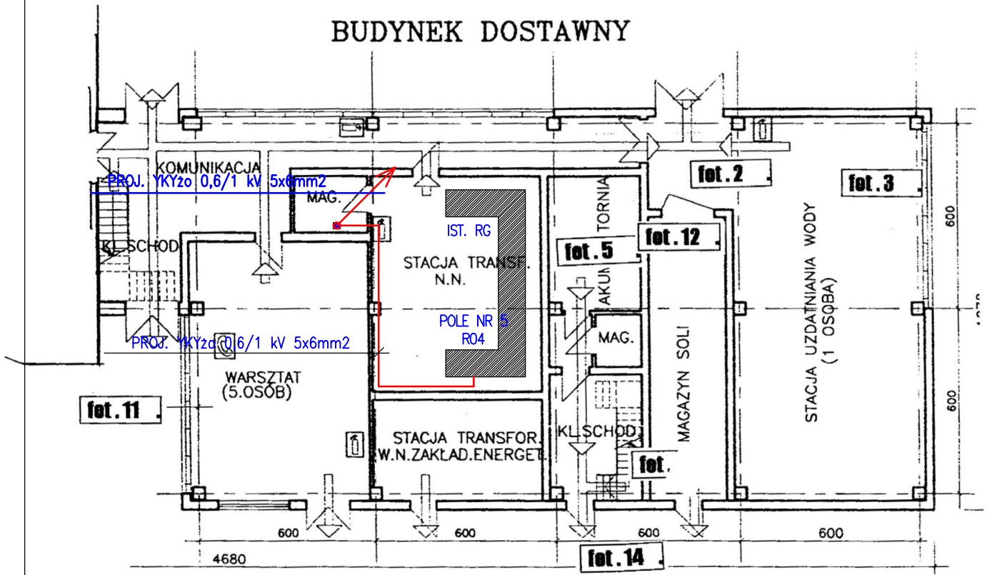
RZUT PRZYZIEMIA - POZ. 0.00
